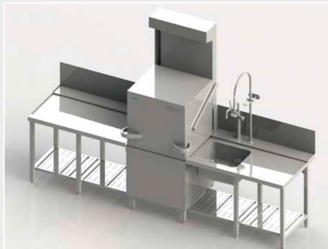
PT-L EnergyPlus Durchlaufrichtung rechts-links
