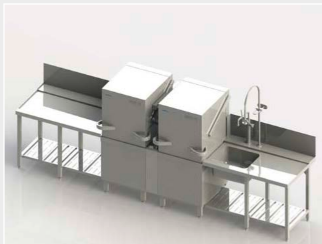
PT-M TwinSet Durchlaufrichtung rechts-links
