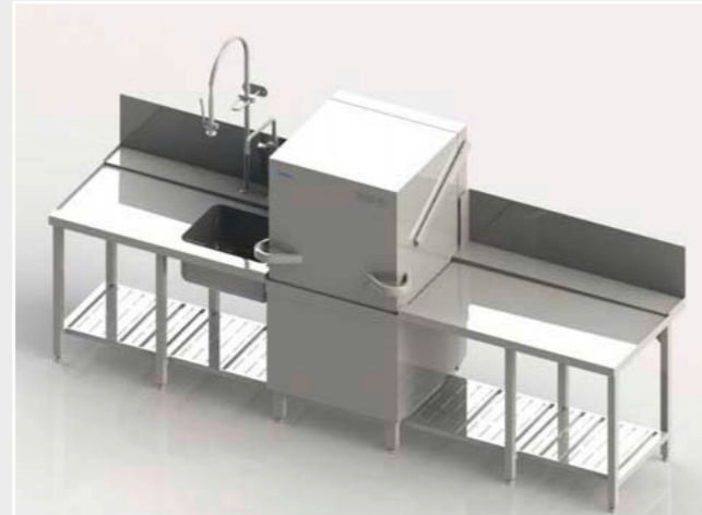
PT-L Durchlaufrichtung links-rechts
